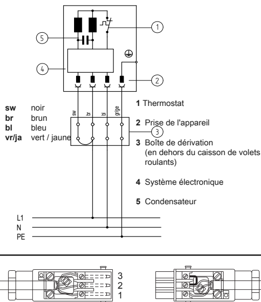
Fig. 5: Plan de câblage RolTop-868 230 V / 50 Hz et pose du câble avec raccord enfichable Hirschmann STAS-3 (avec pont)
