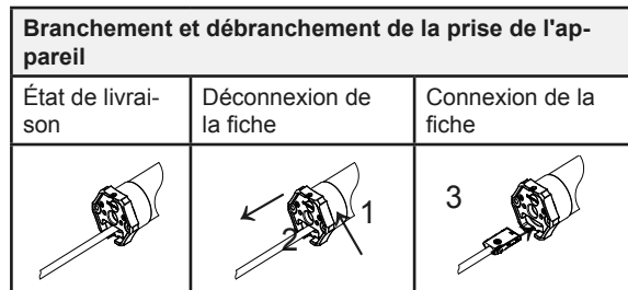
Fig. 4: Branchement et débranchement de la prise de l'appareil
